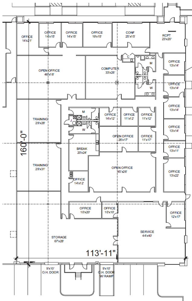
Suite Plan
